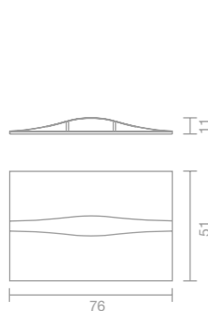
ART. 4500 Applique / Wall lamp Applique / Wandleuchte 76 cm - 29''92 H.51 cm - H.20''07 1x26W - Gx24 -
