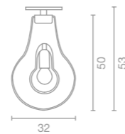
ART. 2743 Plafoniera / Ceiling lamp Plafonnier / Deckenleuchte
