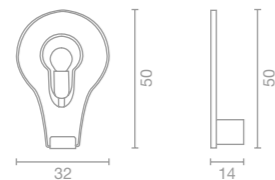
ART. 2745 Applique / Wall lamp Applique / Wandleuchte
