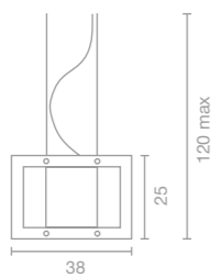
ART. 0460 Sospensione / Suspension Suspension / Hängeleuchte 38x11 cm - 14"96x4"33 H.25 cm - H.9"84 H.120 cm max - H.47"24 max 1x70W - E27 -
